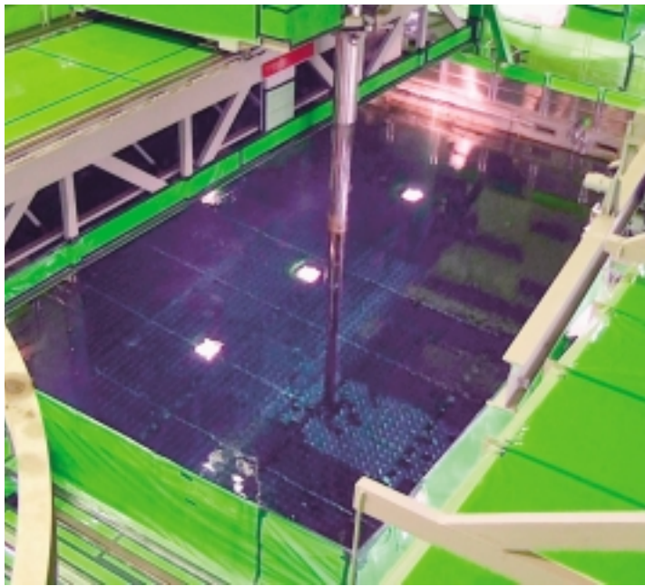
使用済燃料プール（中部電力株式会社より提供）
