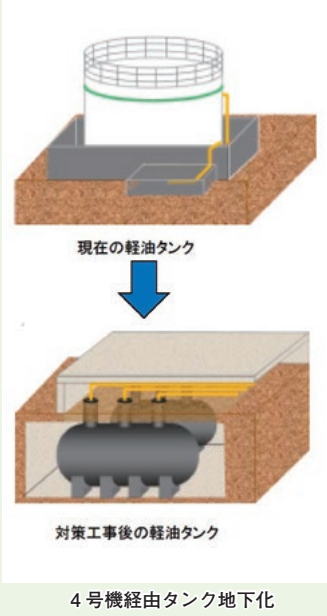
4号機經由タンク地下化
