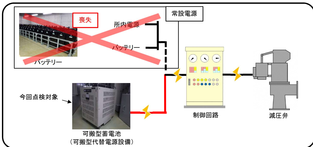
可搬型代替電源設備の概略図
