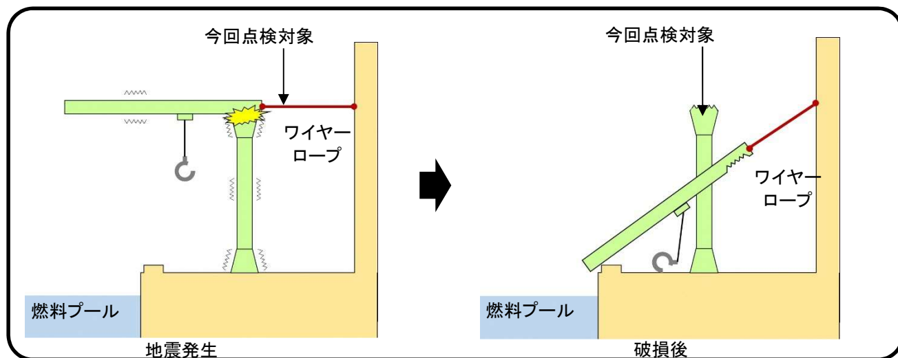
燃料プールを損傷させる可能性のある設備に施したワイヤーロープ 概略図
