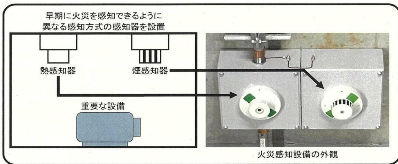
火災感知設備の設置に関する概略図
