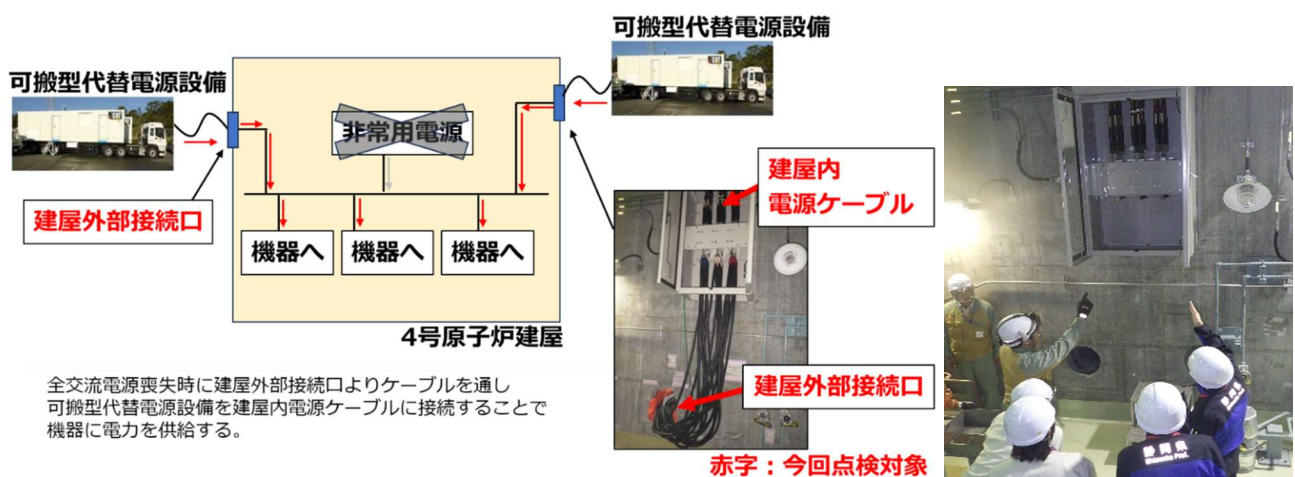
代替電源設備の電源系統概略図
