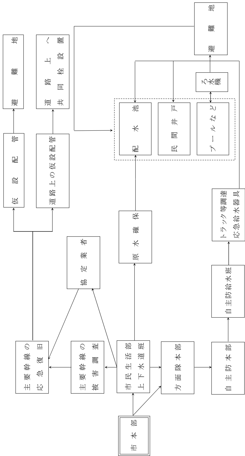
17-1 応急給水活動フローチャート
